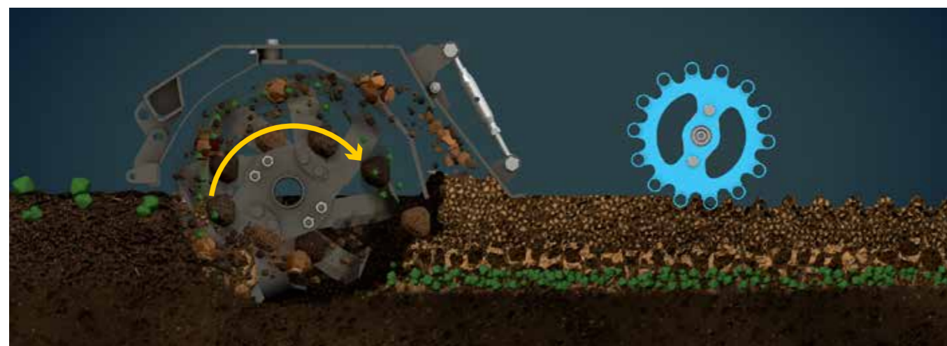
▲ Arbeitsweise der Umkehrfräse, also der Frässtelle, die entgegen der Fahrtrichtung rotiert. Rückstände werden eingefräst.
